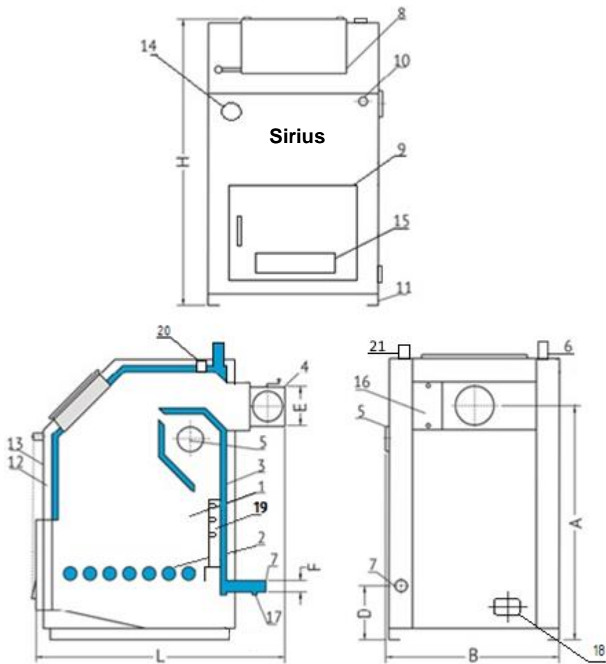
Рис. 1 Вид котла Sirius KB
