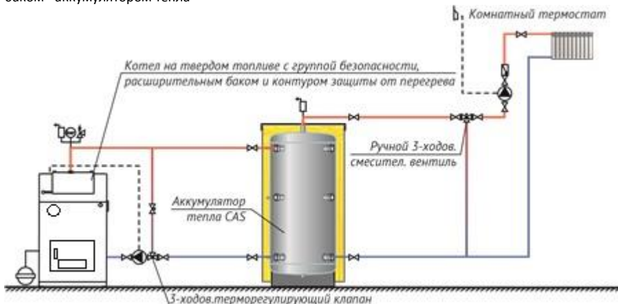
Рис.6 Принципиальная гидравлическая схема соединения котла Sirius в закрытой системе отопления с баком - аккумулятором тепла
